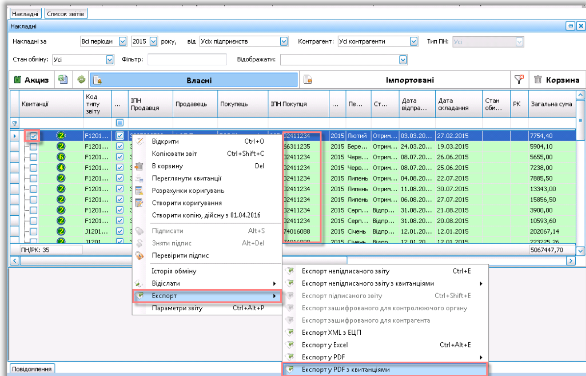
Виклик функції експорту запису у pdf формат з квитанціями
